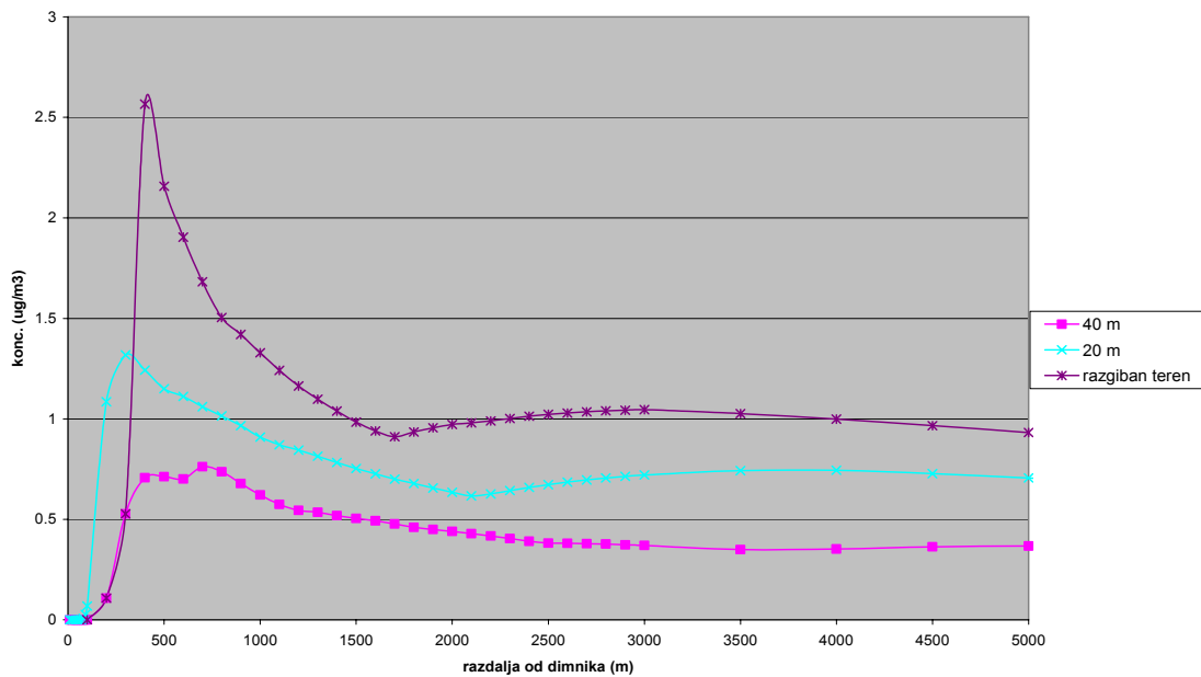
Slika 10.8: Maksimalna 1 urna koncentracija svinca iz Steklarne Rogaška v odvisnosti od efektivne višine dimnika. Izračuni so bili narejeni nad ravnim terenom in različnimi efektivnimi višinami (20 in 40 m) ter dejansko višino dimnika (40 m) in terena v okolici. Rezultati so izračunani z modelom Screen 3
